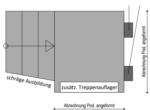
Fingerauflager
