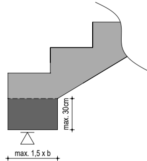
Aufstandssockel
